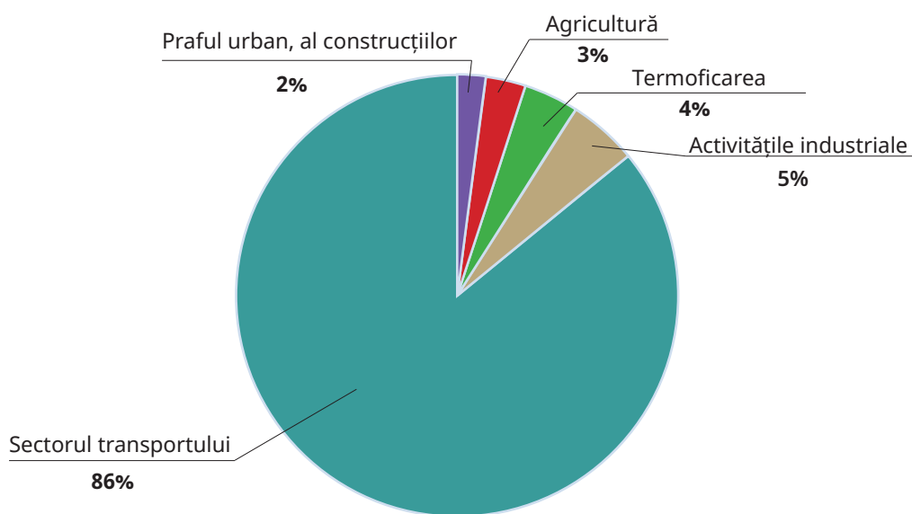
Fig.5. Surse de poluare a aerului în zonele urbane ale Moldovei 9
